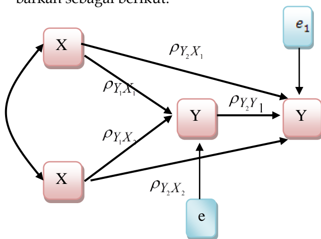
Gambar 2. Jalur Antarvariabel
